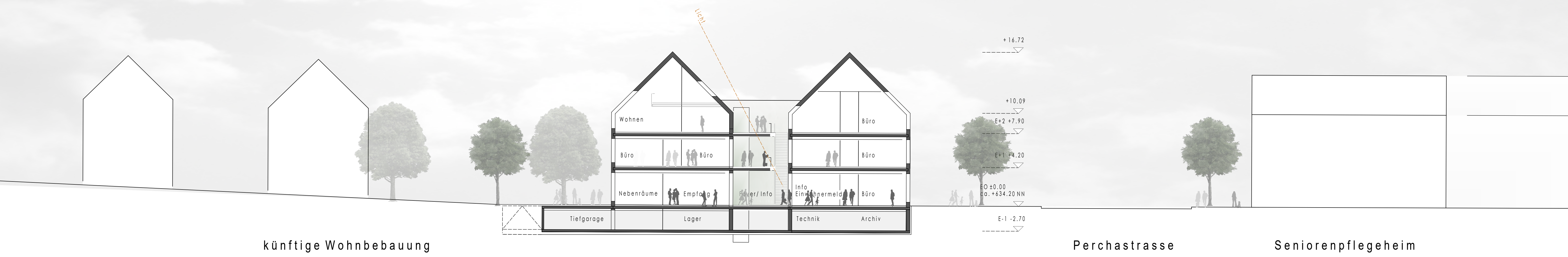
SCHNITT A - A M 1 . 200
